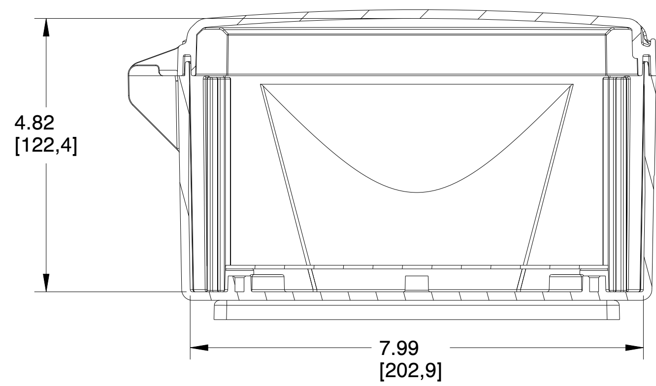
SECTION A-A
