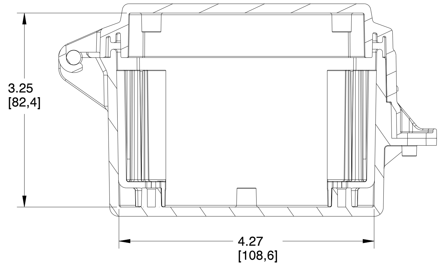
SECTION A-A
